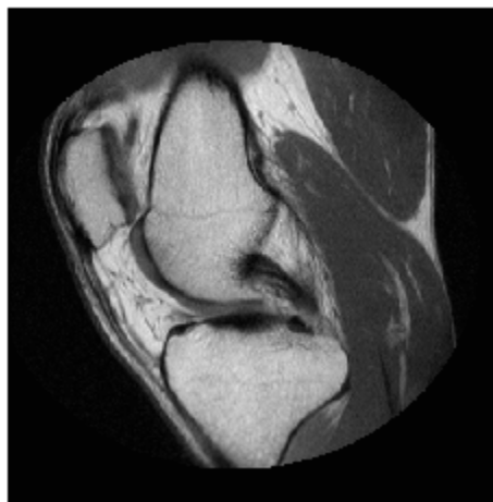
B16bitUniq: N = 448
